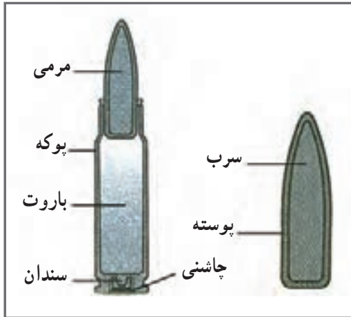
اجزای فشنگ جنگی معمولی
